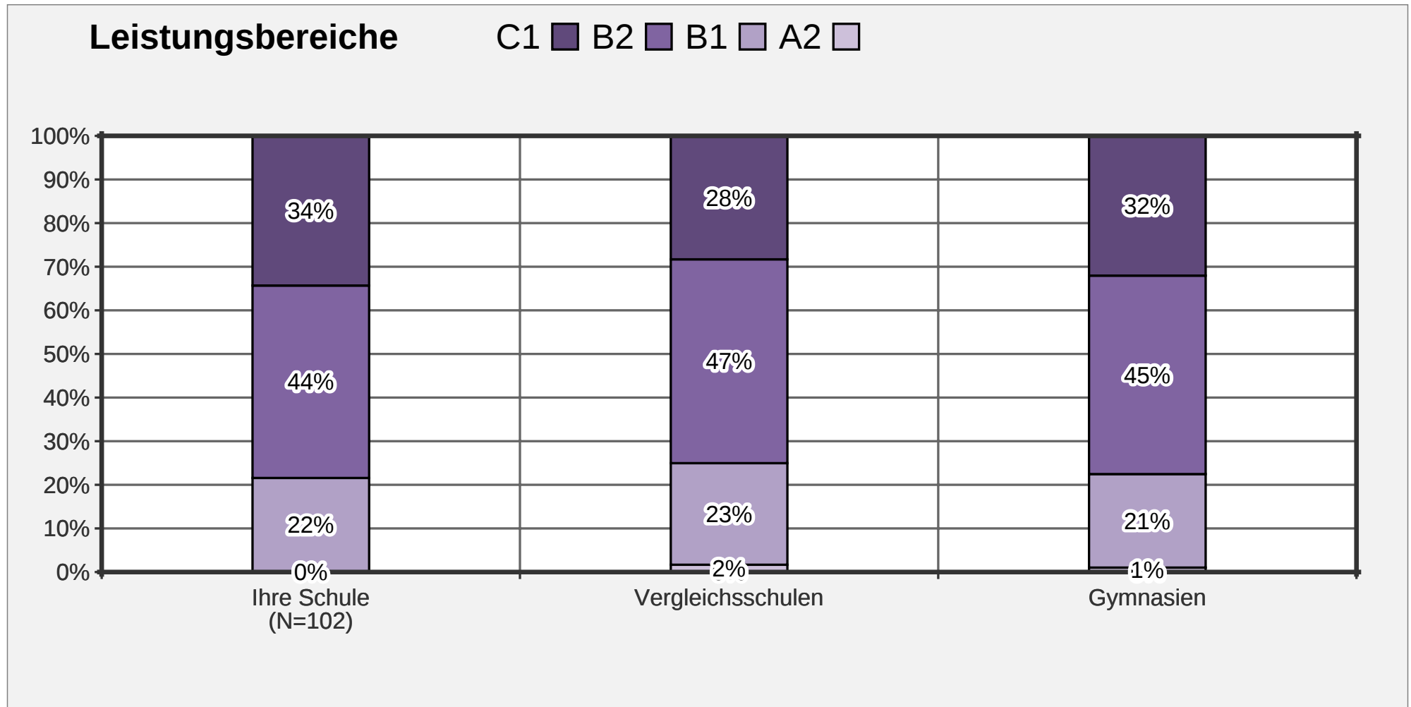
Abbildung 8: Englisch-Hörverstehen: Leistungsverteilungen
