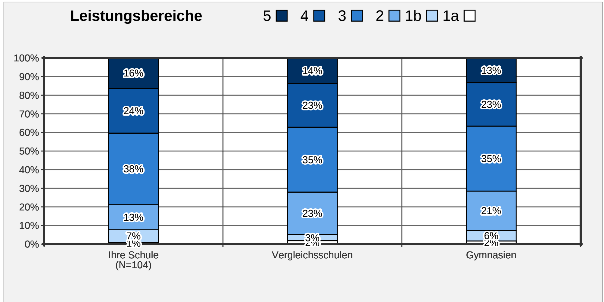
Abbildung 10: Mathematik - Leistungsverteilungen
