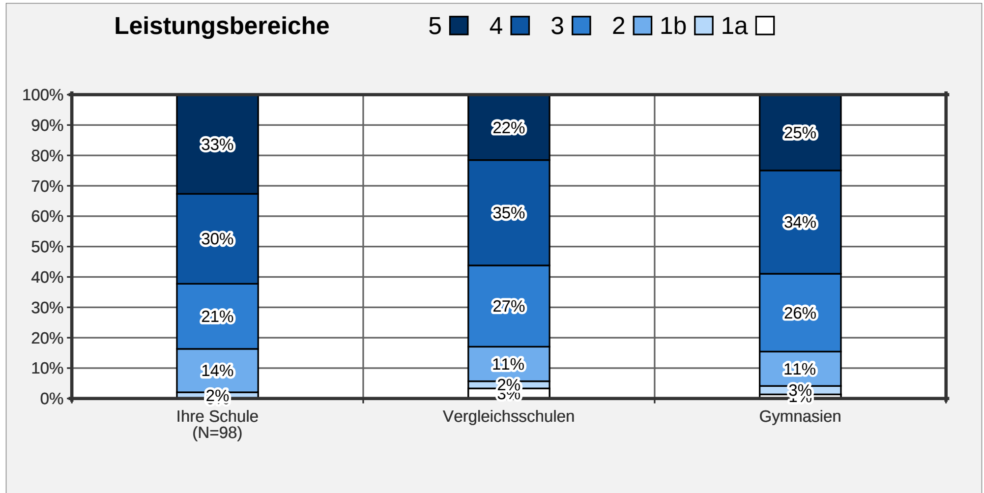
Abbildung 4: Deutsch-Hörverstehen: Leistungsverteilungen
