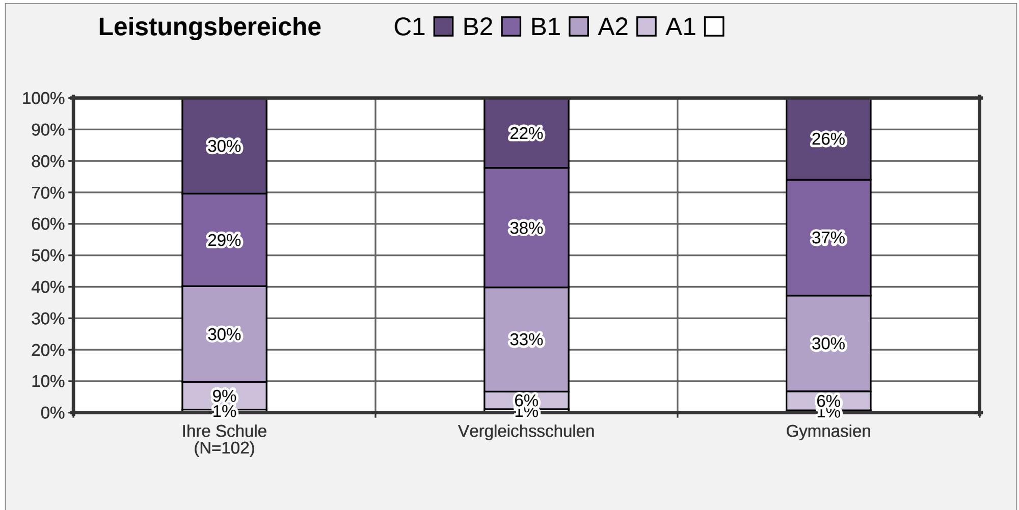
Abbildung 6: Englisch-Leseverstehen - Leistungsverteilungen
