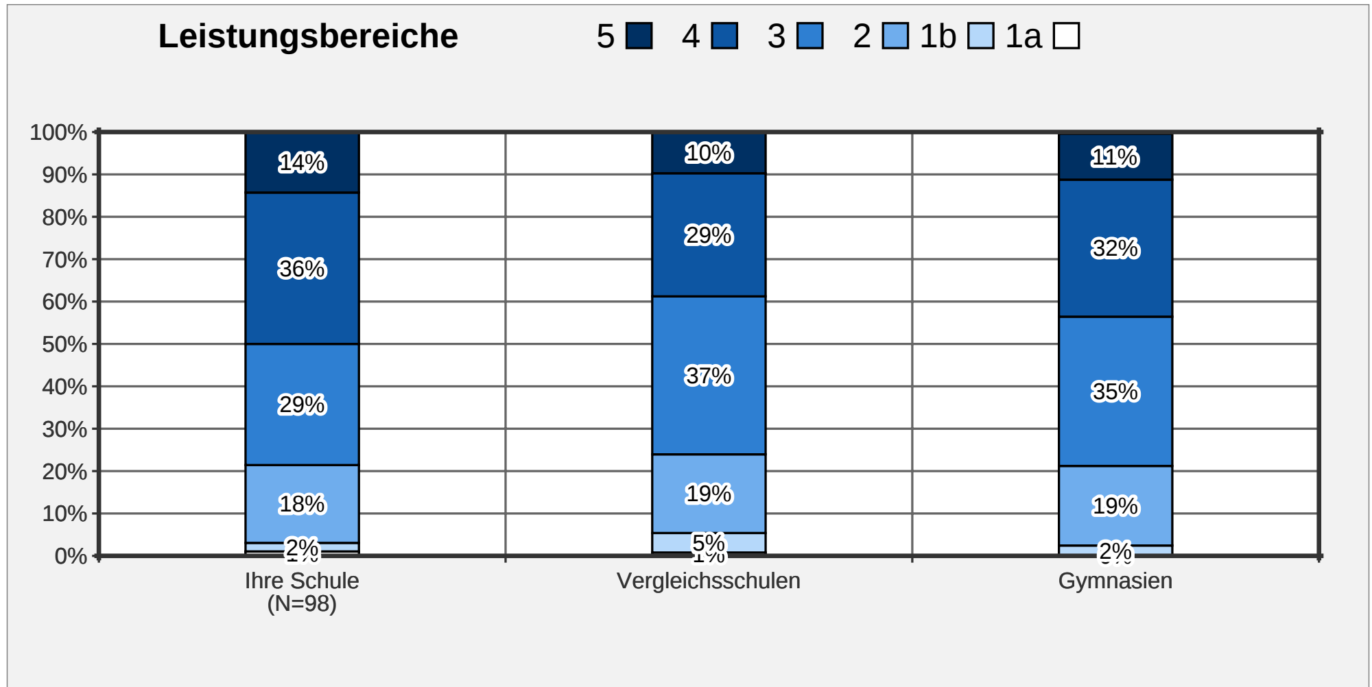
Abbildung 2: Deutsch-Leseverstehen - Leistungsverteilungen
